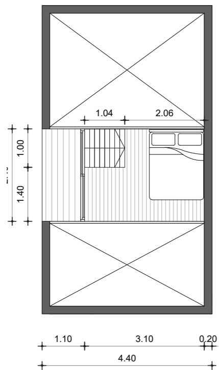
PLANTA ALTA
