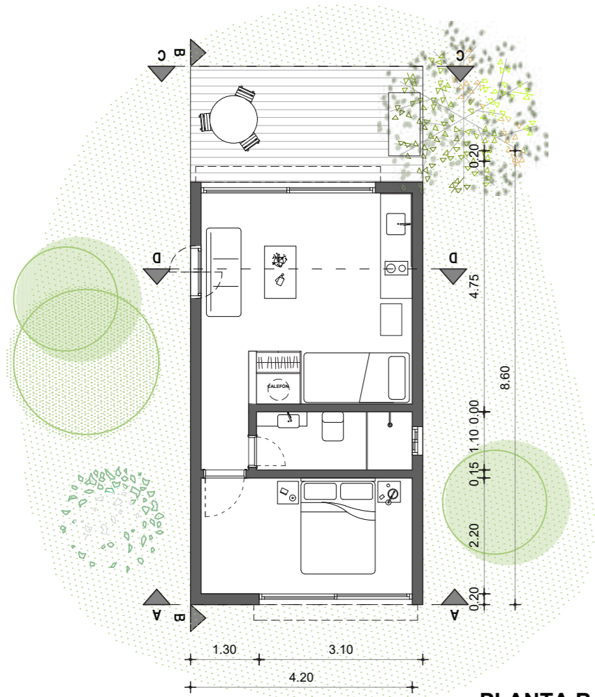
PLANTA BAJA
